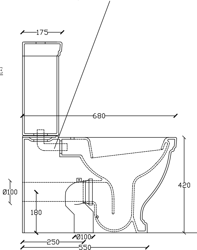
Vista laterale Lateral View Vista lateral Vue latérale
