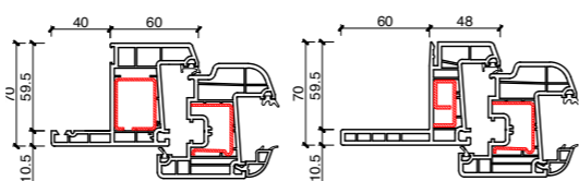
Telaio restauro al.40 Anta Z Arrotondata
