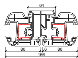
Nodo Centrale
