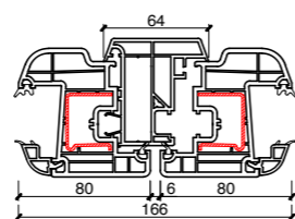
Nodo Centrale
