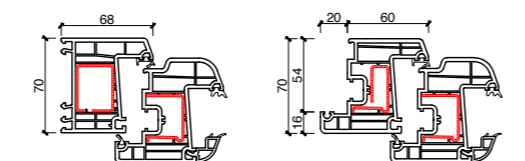
Telaio L - Anta Z Arrotondata
