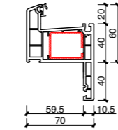
Telaio restauro aletta 40
