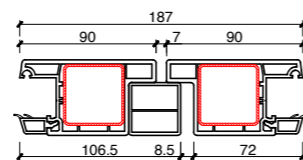
Nodo centrale persiana
