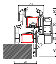
Telaio restauro 40 - Anta Z arrotondata
