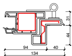
Anta e Telaio Persiana
