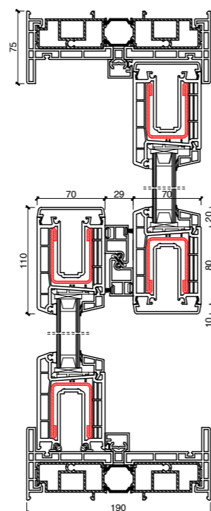
Alzante Sezione Orizzontale
