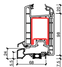
Soglia Alluminio Taglio Termico con anta portone
