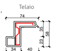
Anta e Telaio Persiana
