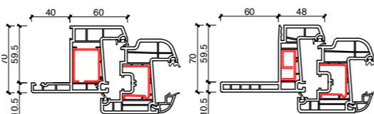
Telaio restauro al.40 Anta Z Arrotondata
