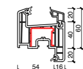
Telaio Z 20
