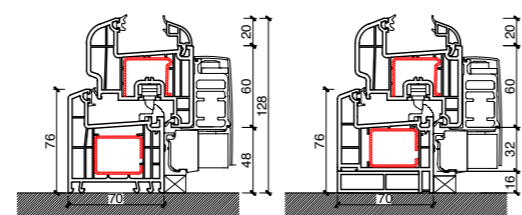
Telaio L 76 - Anta Z arrotondata
